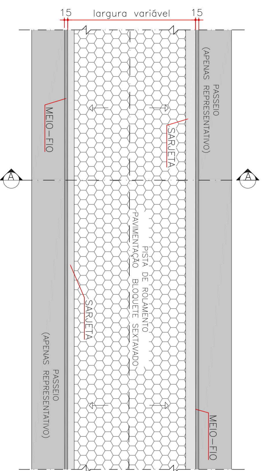
PLANTA PAVIMENTAÇÃO SEM ESCALA
