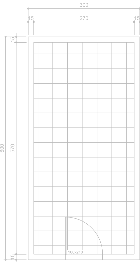
PLANTA DEPOSITO ESC:1/50
