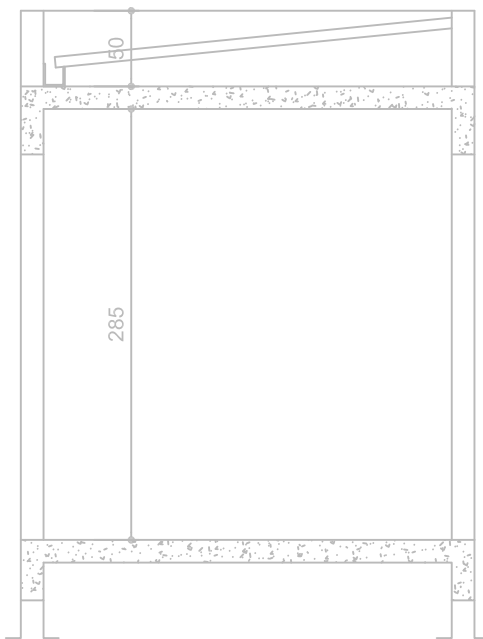
CORTE TRANSVERSAL DEPOSITO ESC:1/50
