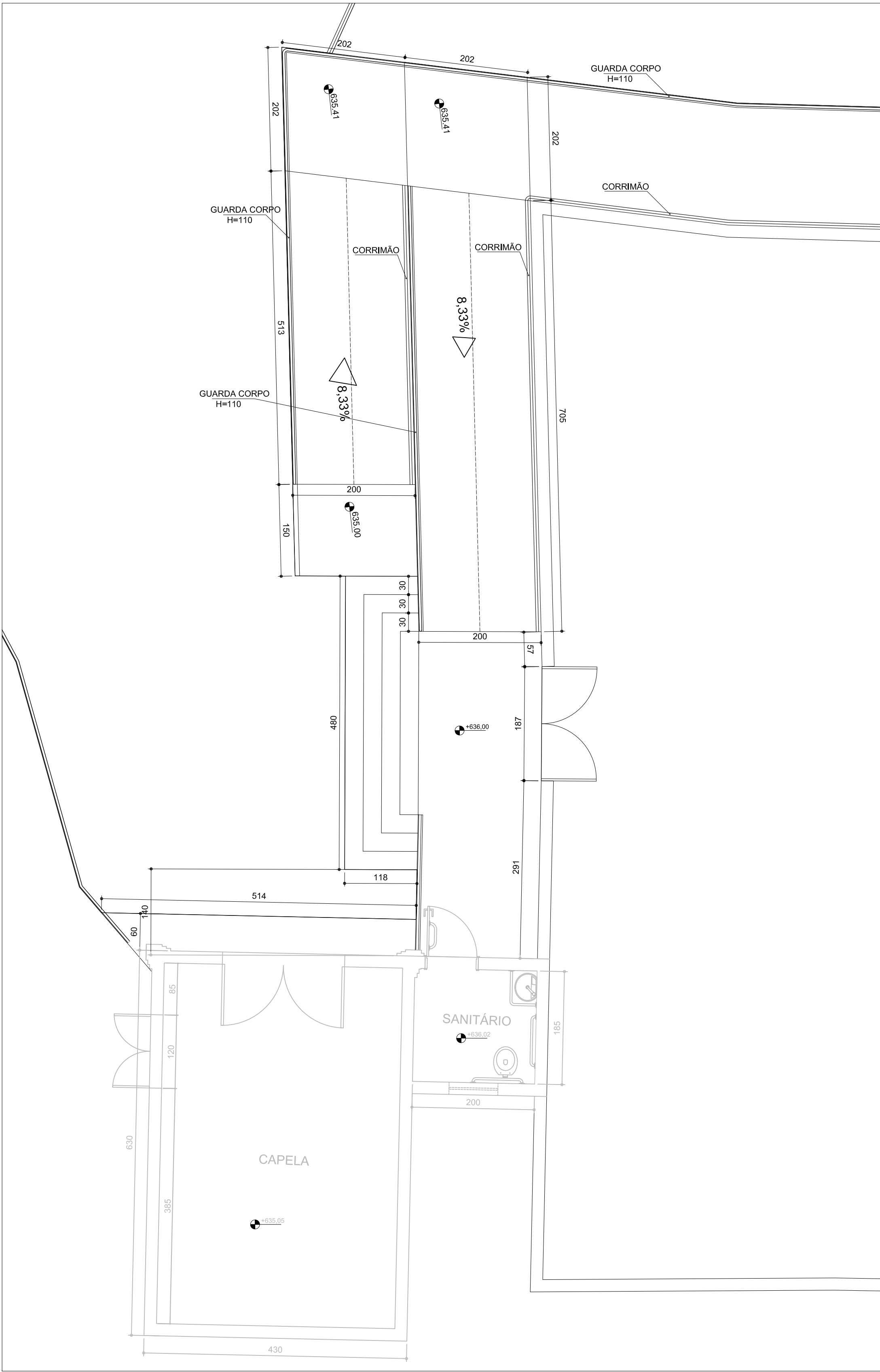
PLANTA RAMPA DE ACESSO ESC:1/50
