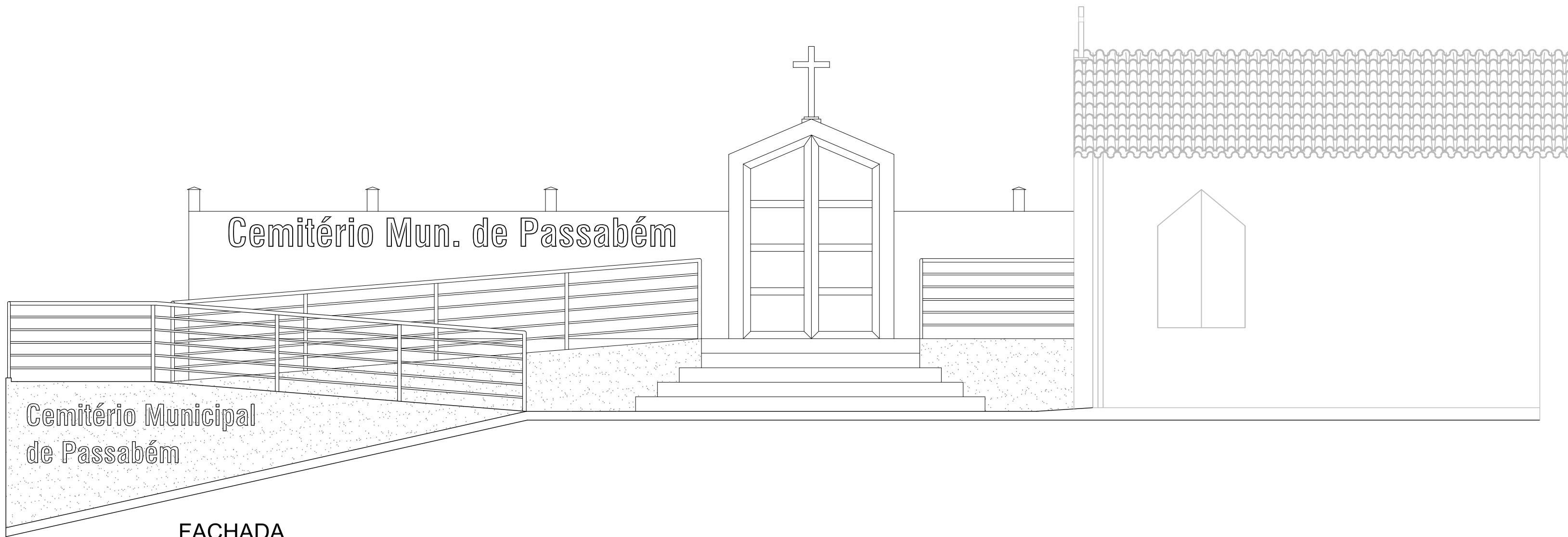
FACHADA RAMPA DE ACESSO ESC:1/50
